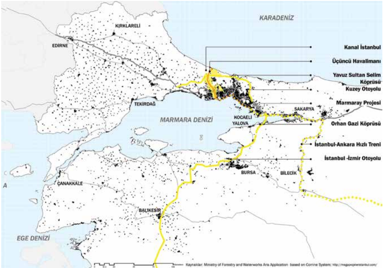
Figür 1: İstanbul ve Marmara Bölgesi ölçeğinde mega projeler ve kentsel alanlar. Kaynak: Özlem Altınkaya Genel, Shifting Scales of Urban Transformation: The Emergence of the Marmara Urban Region between 1990 and 2015 , yayımlanmamış doktora tezi, Harvard Graduate School of Design, 2016; TC Orman ve Su İşleri Bakanlığı Corine Projesi; https://megaprojeleristanbul.com/
