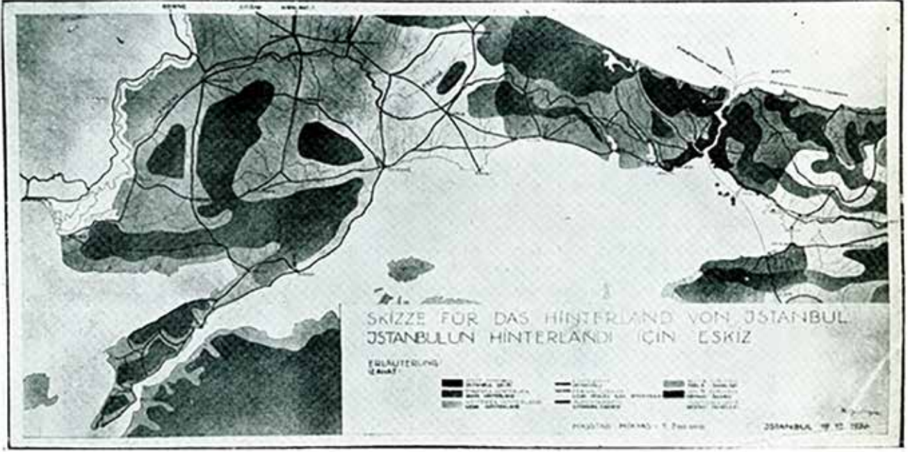
Figür 5: Wagner Planı: İstanbul'un hinterlandı için eskiz.
