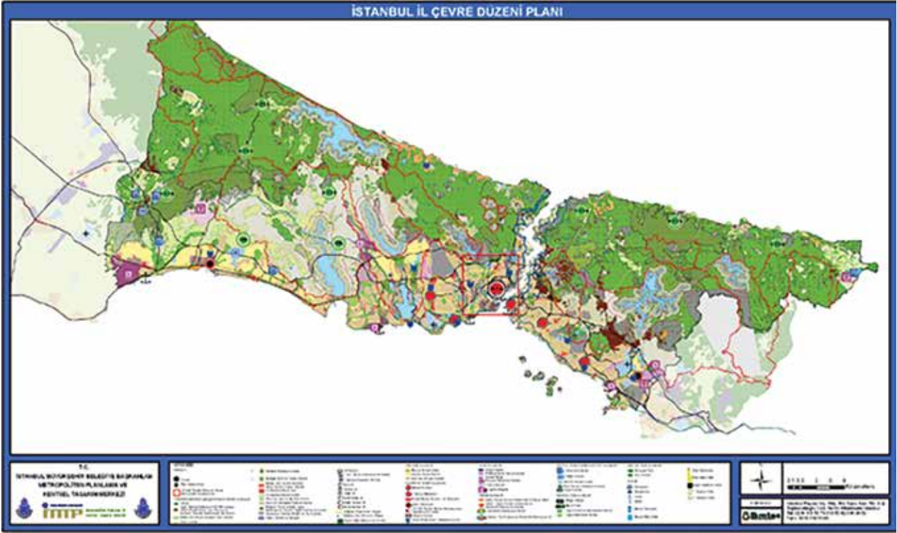
Figür 7: 1/100.000 Ölçekli İstanbul İl Çevre Düzeni Planı.
