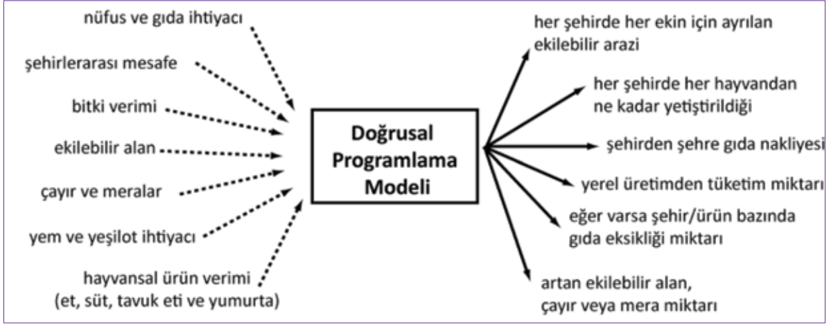
Şekil 1: Doğrusal programlama modeli girdi ve çıktılar
