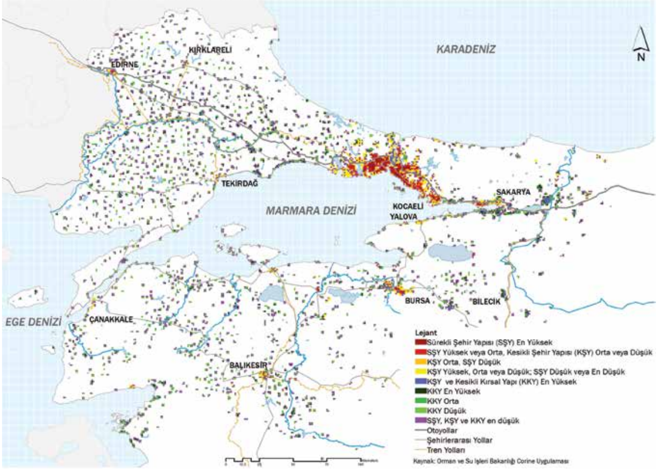
Figür 3: Marmara Bölgesi'nde 2006 yılına ait kentsel ve kırsal alan katmanlaşması. Kaynak: Orman ve Su İşleri Bakanlığı Corine Projesi.
