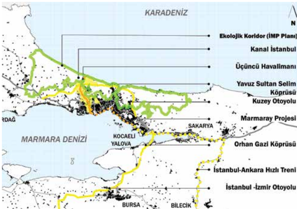
Figür 2: Mega projeler ve 1/100.000 ölçekli İstanbul Çevre Düzeni Planı'nda tanımlanan ekolojik koridor. Kaynak: Altınkaya Genel, a.g.e., 2016; TC Orman ve Su İşleri Bakanlığı Corine Projesi; https://megaprojeleristanbul.com/
