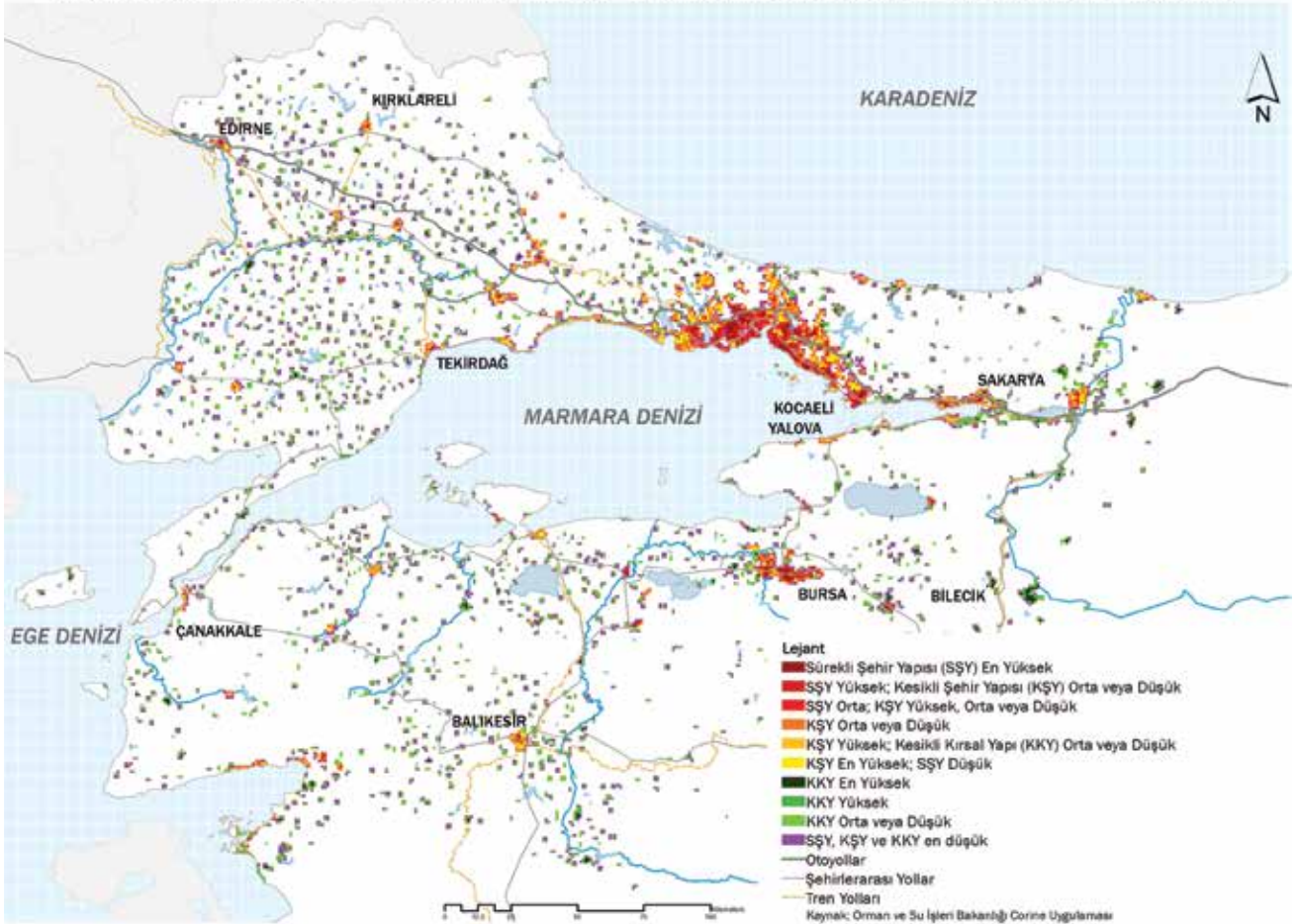
Figür 4: Marmara Bölgesi'nde 2012 yılına ait kentsel ve kırsal alan katmanlaşması. Kaynak: Orman ve Su İşleri Bakanlığı Corine Projesi.
