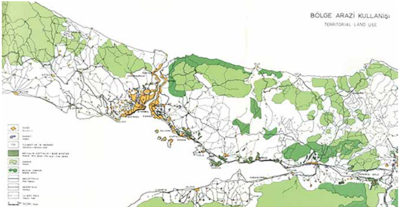
Figür 6: Doğu Marmara Ön Planı: Bölge arazi kullanışı.
