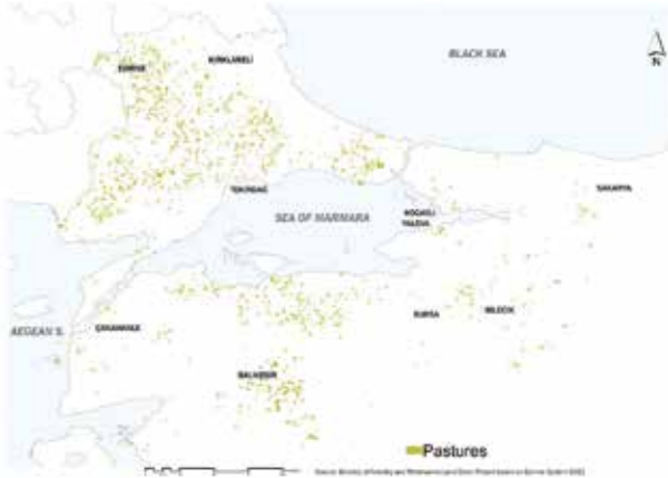
Figür 8: Marmara Bölgesi’nde 2012 yılına ait mera alanları arazi örtüsü dağılımı. Kaynak: Orman ve Su İşleri Bakanlığı Corine Projesi.
